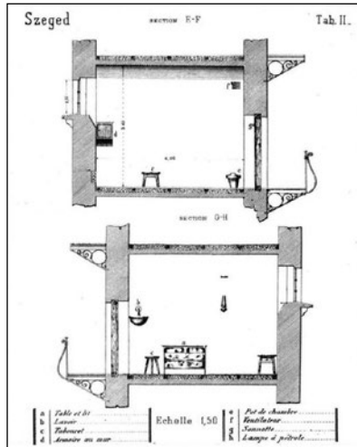
2. kép: Zárka keresztmetszete 22
