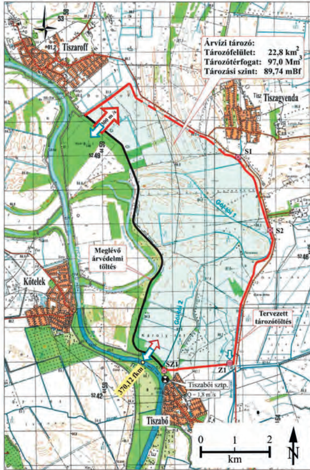
6. ábra A Tiszaroffi árvízi (VTT) tározó átnézeti helyszínrajza (Országos Vízügyi Főigazgatóság, http://www.vizugy.hu/uploads/files/Tiszaroff%20.jpg ) Figure 6 Plan view of the flood storage reservoir (VTT) at Tiszaroff (General Directorate of Water Management, http://www.vizugy.hu/uploads/files/Tiszaroff%20.jpg )
