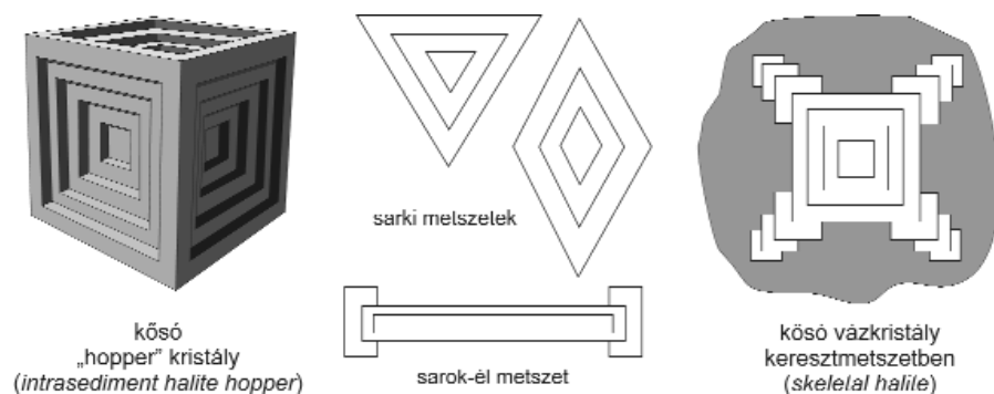
3. ábra. A kősó vázkristályok morfológiája és jellemző mikroszkópi metszetei WARREN (2006) nyomán módosítva
