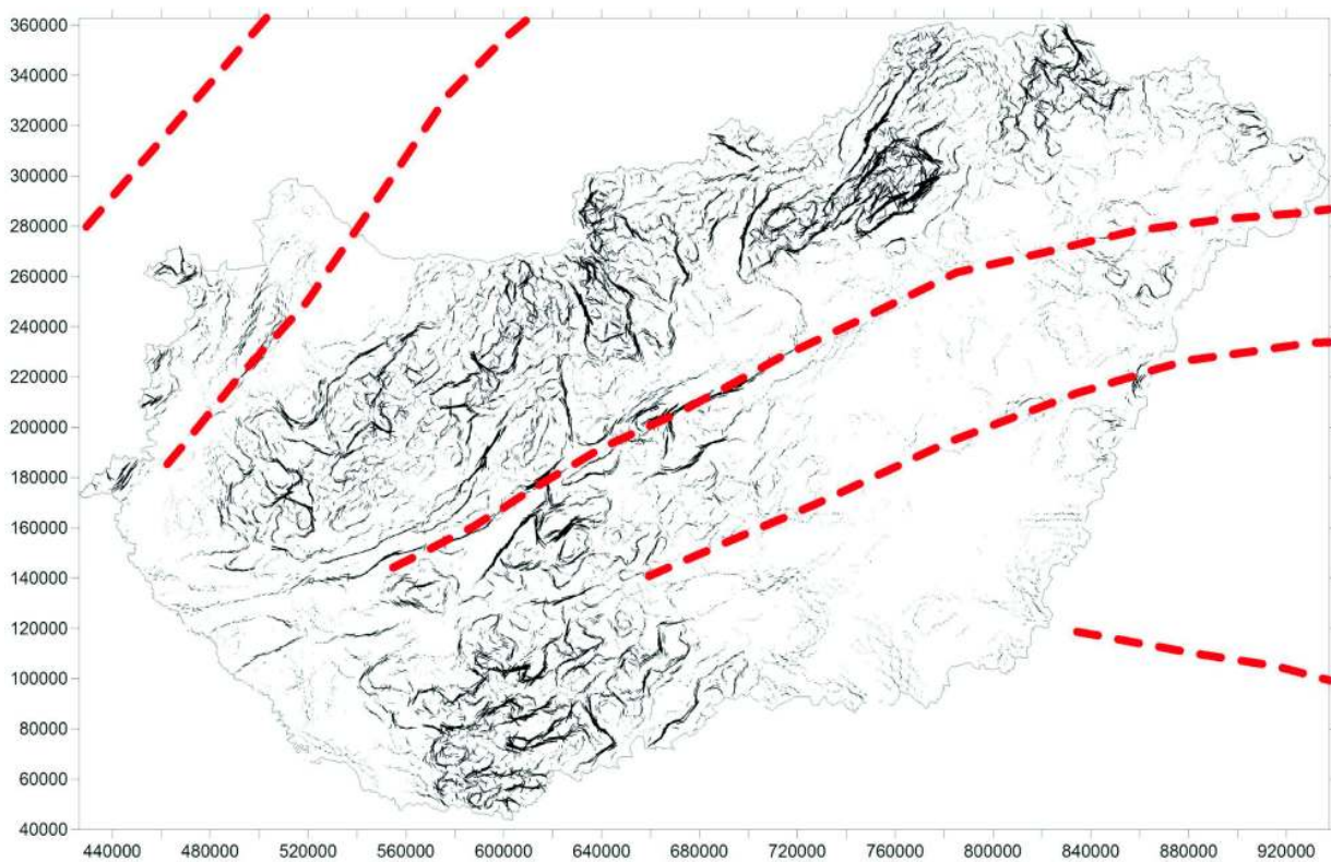
19. ábra. Gravitációs hatóperemek az országos adatrendszerből (Kiss 2006) és kéregszerkezeti vonalak a régió adatai alapján Figure 19. Gravity edge detections of Hungary (Kiss 2006) and simplified lineaments of Carpathian-Pannonian Region
