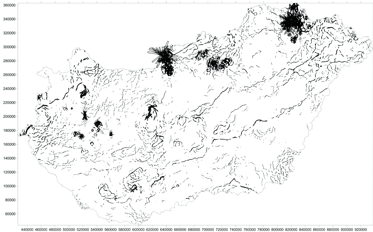
16. ábra. Digitális feldolgozásból nyert mágneses hatóperemek Magyarország területén (Kiss 2013a)
