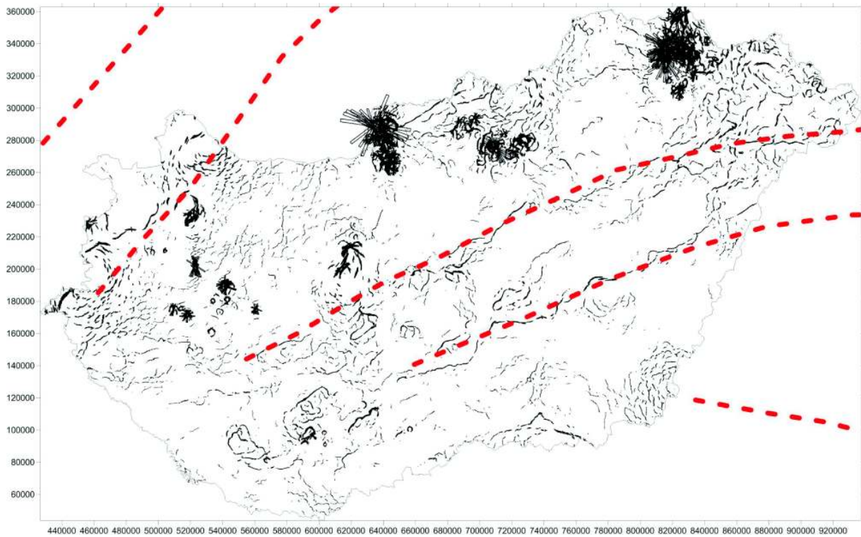
18. ábra. Mágneses hatóperemek az országos adatrendszerből (Kiss 2013a) és kéregszerkezeti vonalak a régió adatai alapján Figure 18. Magnetic edge detections of Hungary and simplified lineaments of Carpathian-Pannonian Region (Kiss 2013)
