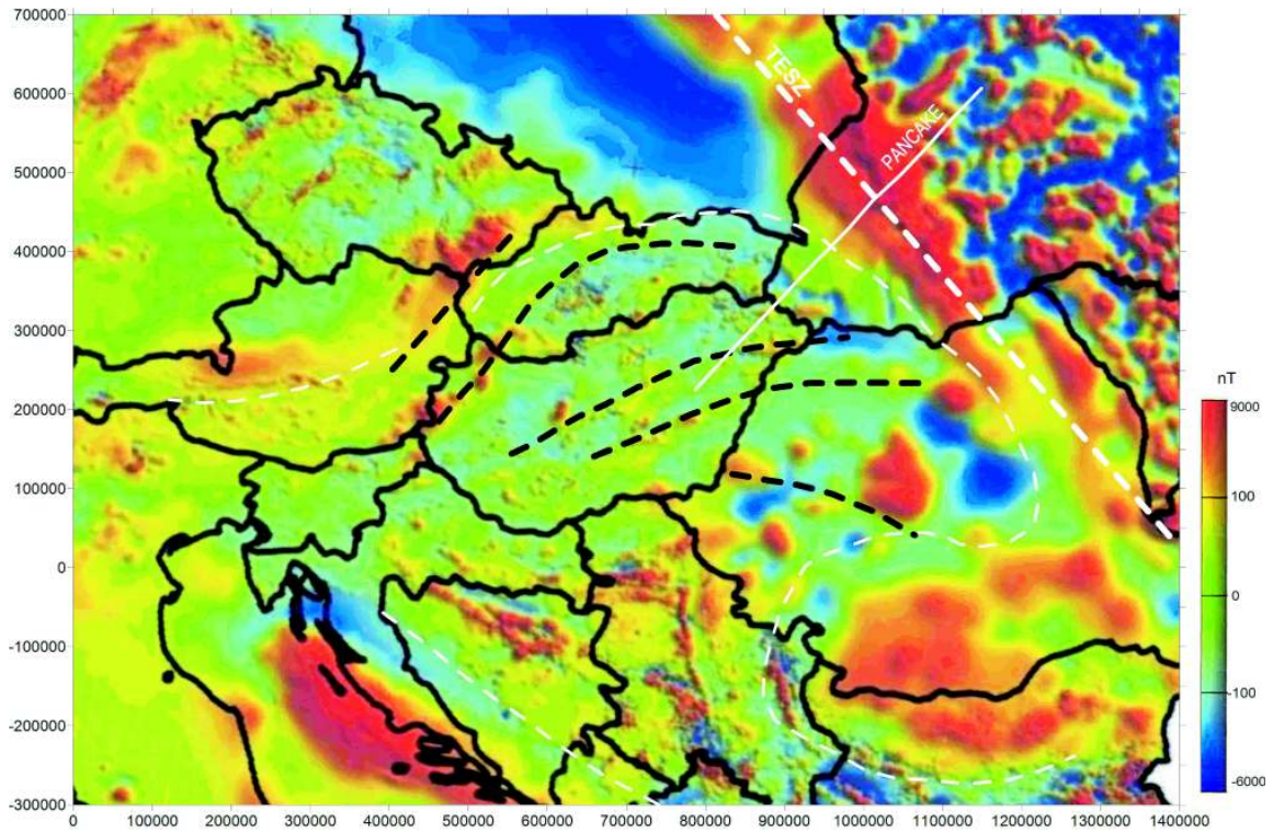
13. ábra. Egyszerűsített lineamensek a Kárpát–Pannon-régió mágneses anomália térképén
