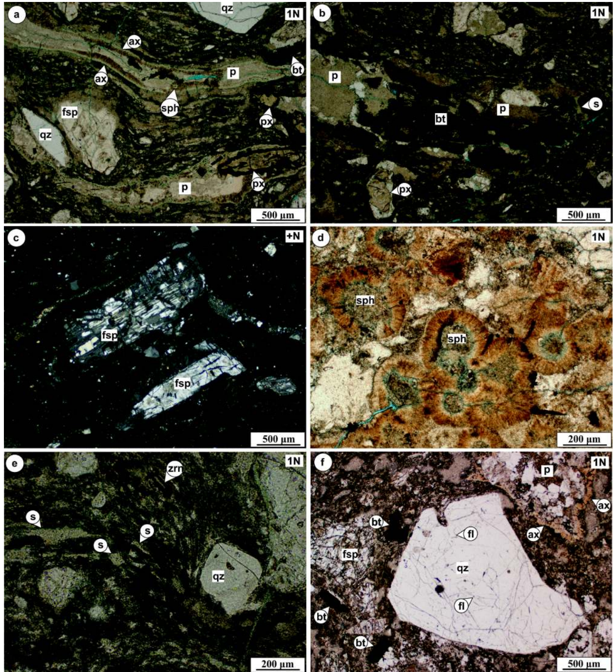
4. ábra. Az eutaxitos szövetű, összesült, kristálygazdag horzsakótartalmú lapillitufa litofáciest bemutató mikrofotók. a) Egymással párhuzamosan futó horzsakóvek axiolitos szegéllyel és belsejükben szferolitokkal, illetve piroxén utáni opak pszeudomorfozák; b) Horzsakóvet kitöltő biotit utáni opak pszeudomorfoza; c) Töredezett földpát fenokristályok az irányított alpanyagban (kétféle megjelenés); d) Szferolitok a kőzet szövetében; e) Irányítottágot hordozó, átalakult üvegszilánkok; f) Félig sajátalakú, szegélye mentén visszaoldott kvarc, töredezett földpát fenokristály és átalakult horzsakó
