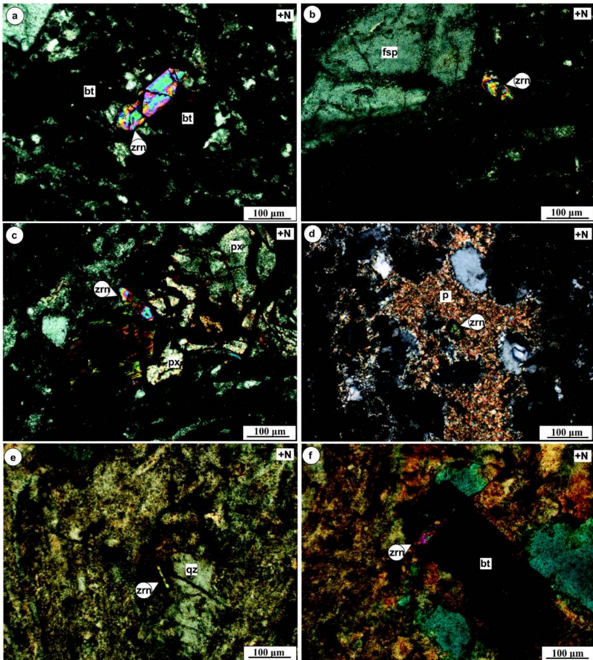
7. ábra. A Győrűfű Riolit felszíni kőzetanyagáról készített cirkon mikrofotók. a) Nagyméretű, az egyik piramisnál törött, sajátalakú cirkon alapanyagban; b) Törött, félig sajátalakú, zónás cirkon alapanyagban; c) Sajátalakú cirkon piroxén utáni opak pseudomorfózában; d) Cirkon átalakult horzsakőben; e) Megnyúlt cirkon kvarc és alapanyag határán; f) Cirkon biotit utáni opak pseudomorfózában
